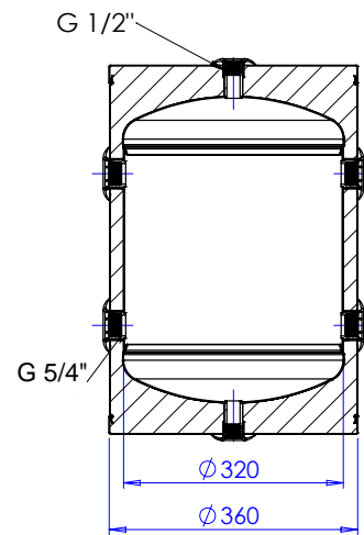
SECTION A-A
